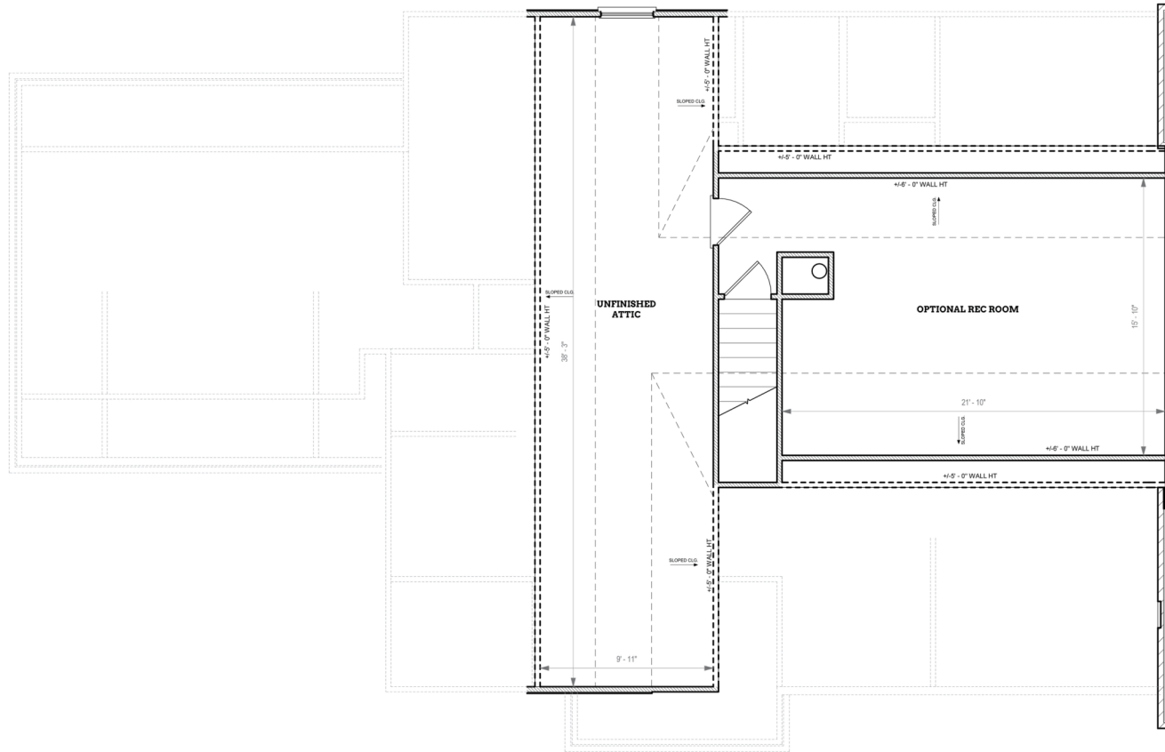
OPTIONAL ATTIC
